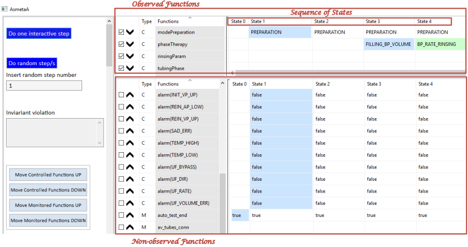
Fig. 2. AsmetaA tool
