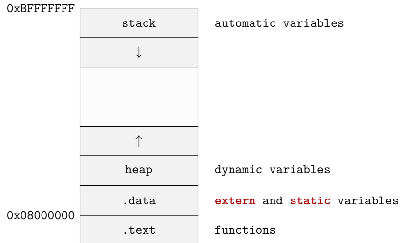
Figura 5 – Layout in memoria di un generico programma C++.
