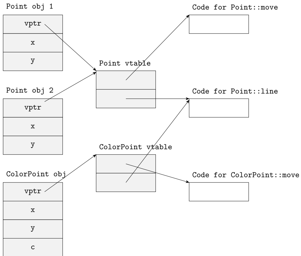
Figura 6 – Rappresentazione del layout in memoria di oggetti con metodi virtual .
